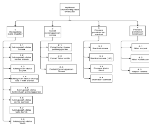
Gambar 6. Diagram Berjenjang
