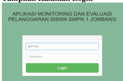
Gambar 13. Halaman Login
