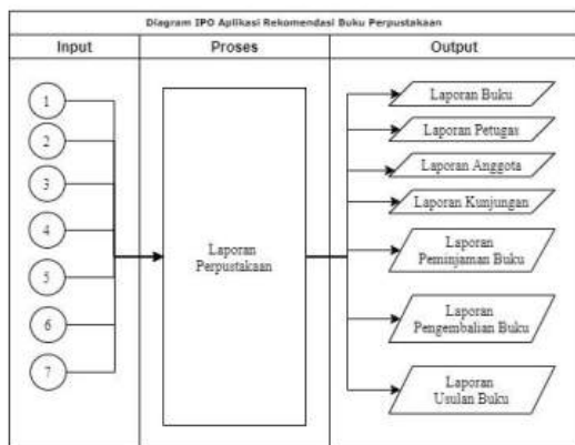
Gambar 3 IPO Lanjutan
