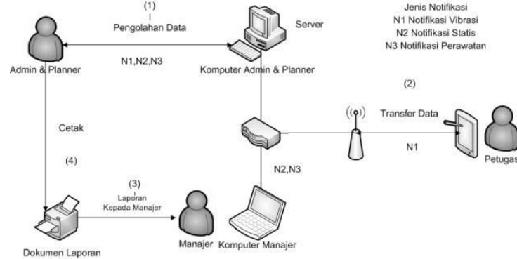
Gambar 2. Solusi Arsitektur aplikasi
