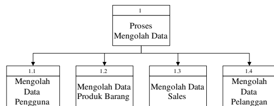
Gambar 5. Diagram berjenjang proses mengolah data
