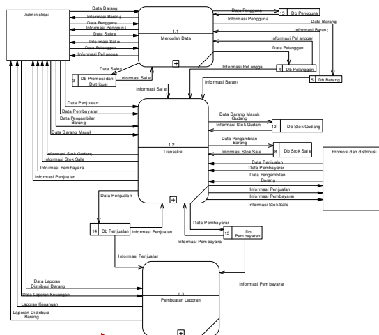
Gambar 8. Data flow diagram level 0 aplikasi
