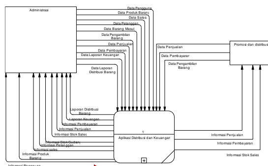
Gambar 3. Context diagram Aplikasi
