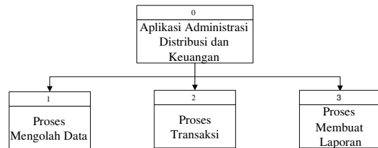
Gambar 4. Diagram berjenjang aplikasi
