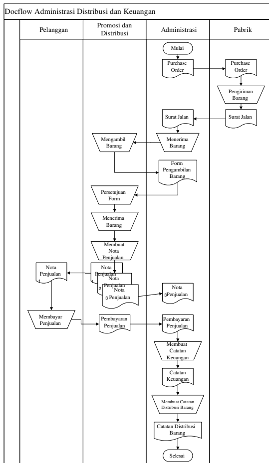
Gambar 1. Document flow Administrasi distribusi dan keuangan
