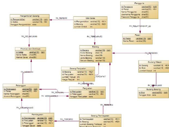
Gambar 13. Model data fisik aplikasi
