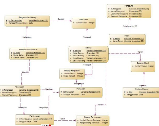
Gambar 12. Model data konseptual aplikasi
