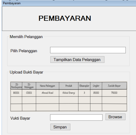
Gambar 10. Halaman Pembayaran
