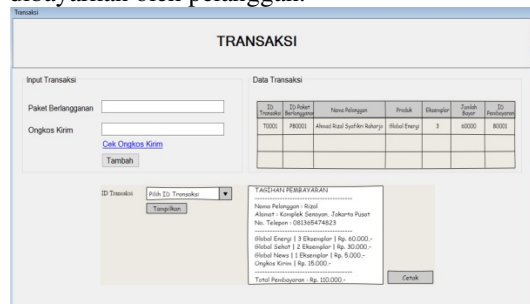
Gambar 9. Halaman Transaksi
