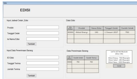
Gambar 7. Halaman Edisi
