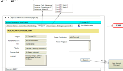
Gambar 13 Perancangan Menu Pengajuan Perpanjangan KP
