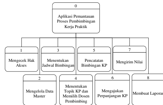
Gambar 3 Hasil Perancangan Diagram Jenjang
