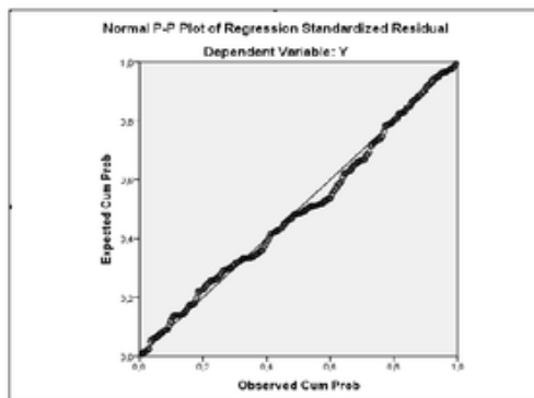
Gambar 6. Grafik P – P Plots
