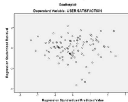
Gambar 7. Grafik Scatterplot
