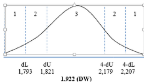
Gambar 8. Daerah Penentuan H_0
