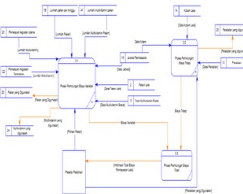
Gambar 6. DFD Level 1 Perhitungan Biaya Pembesaran Ikan Lele
