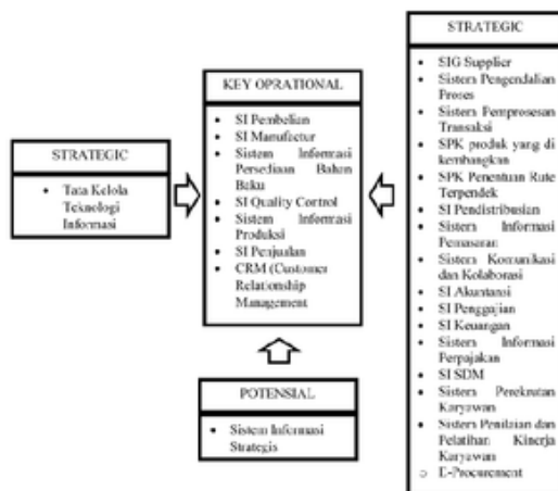
Gambar 6. Pemetaan McFarlan
