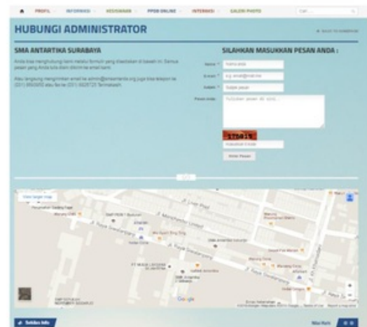
Gambar 11. Form Kontak
