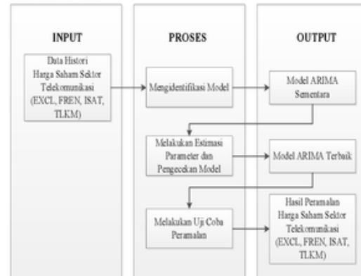
Gambar 1 Blok Diagram Analisis Peramalan Harga Saham Menggunakan Metode Box-Jenkins ARIMA
