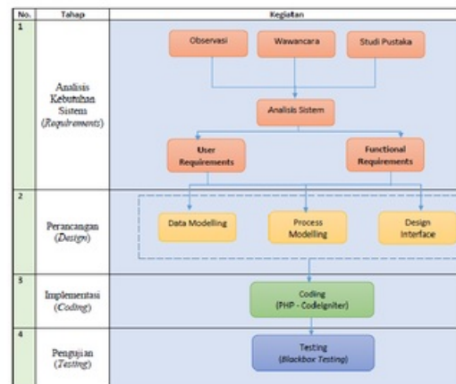
Gambar 1. Tahapan Analisis dan Perancangan Sistem
