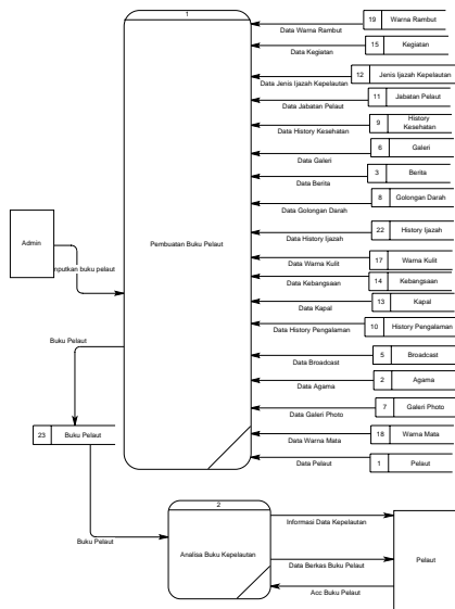
Gambar 10 DFD Level 1 Subproses Administasi Kepelautan
