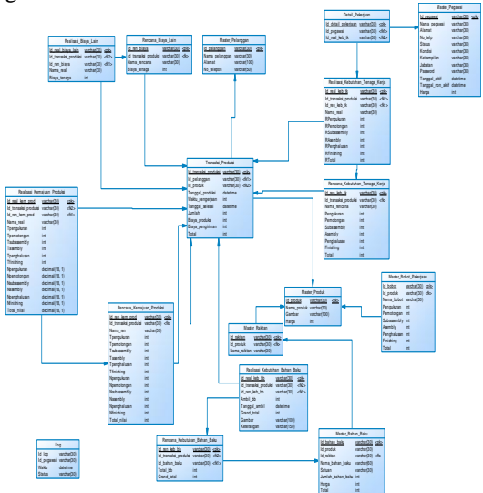
Gambar 10 PDM Sistem Informasi Perencanaan dan Pengawasan Proses Produksi
