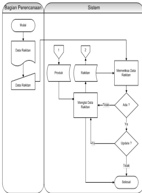
Gambar 3 System Flow Mengolah Data Master Rakitan
