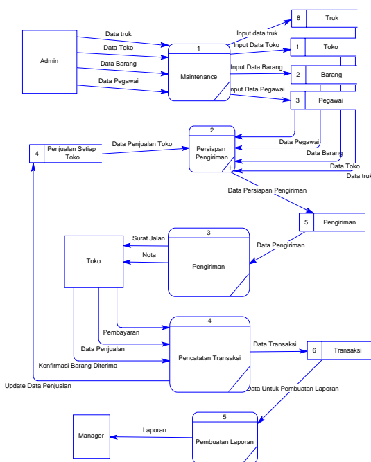
Gambar 3 DFD Level 0 Sistem
