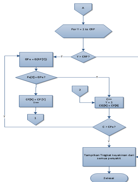
Gambar 2. Flowchart Kombinasi Nilai CF Gejala
