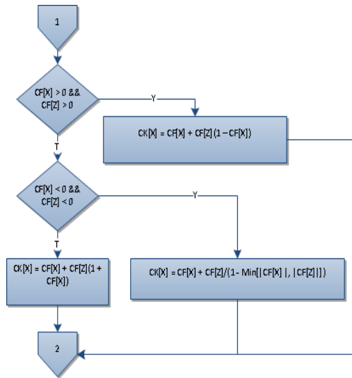
Gambar 3. Flowchart Lanjutan Kombinasi Nilai CF Gejala
