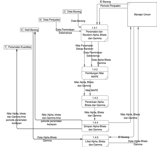
Gambar 11. Proses Penentuan Alpha, Beta dan Gamma.
