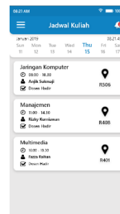
Gambar 18 Jadwal Kuliah
