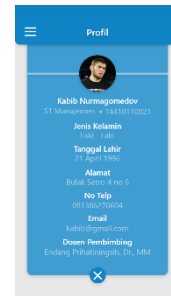
Gambar 28 Halaman Profil
