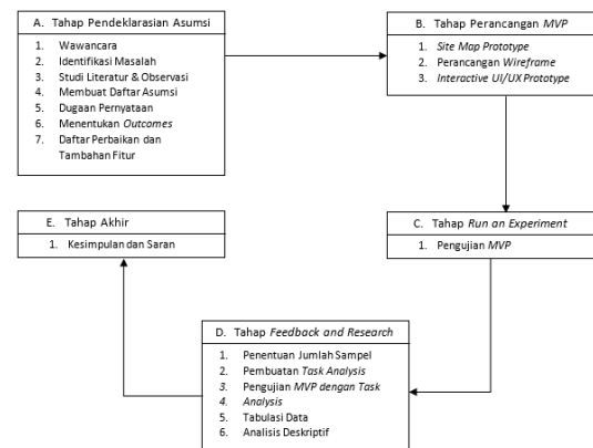
Gambar 2 Metodologi Penelitian
