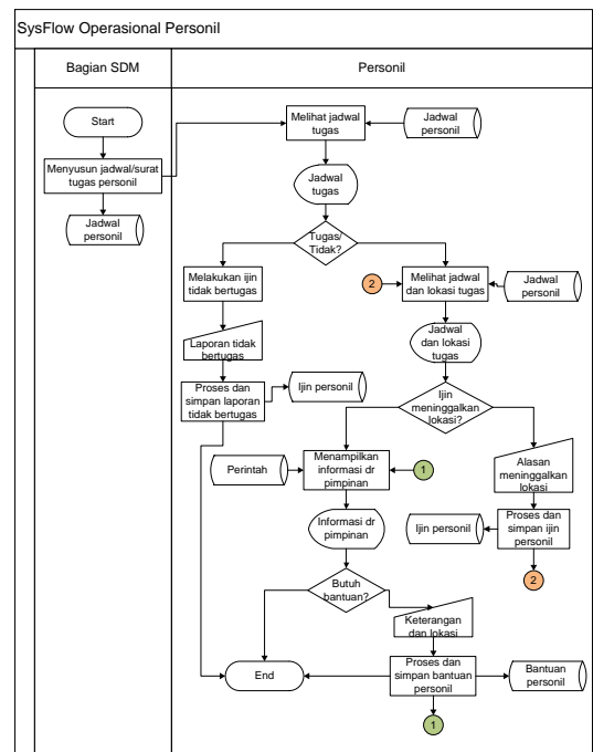
Gambar 5 Sysflow oprasional personil
