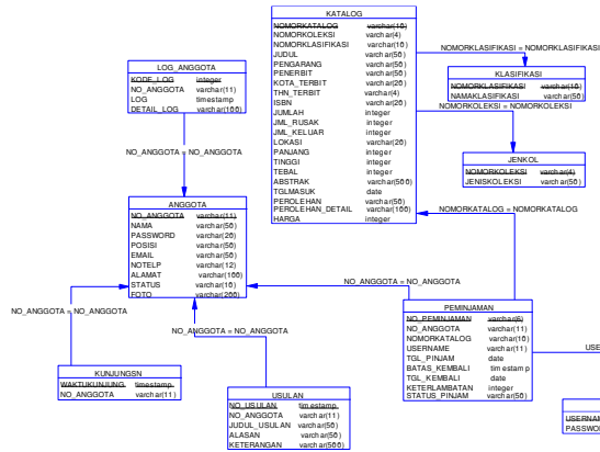
Gambar 11 PDM Sistem Informasi Perpustakaan
