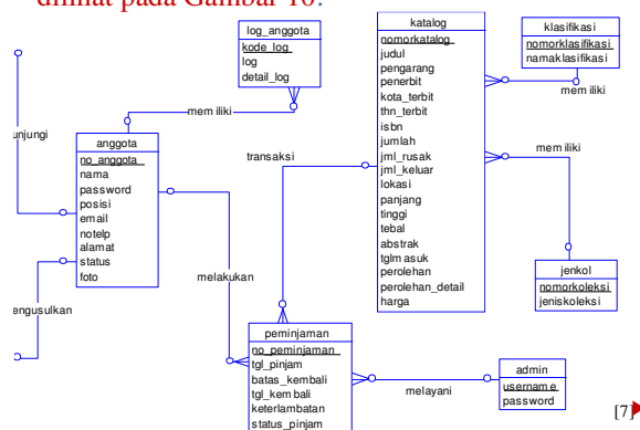
Gambar 10 CDM Sistem Informasi Perpustakaan
