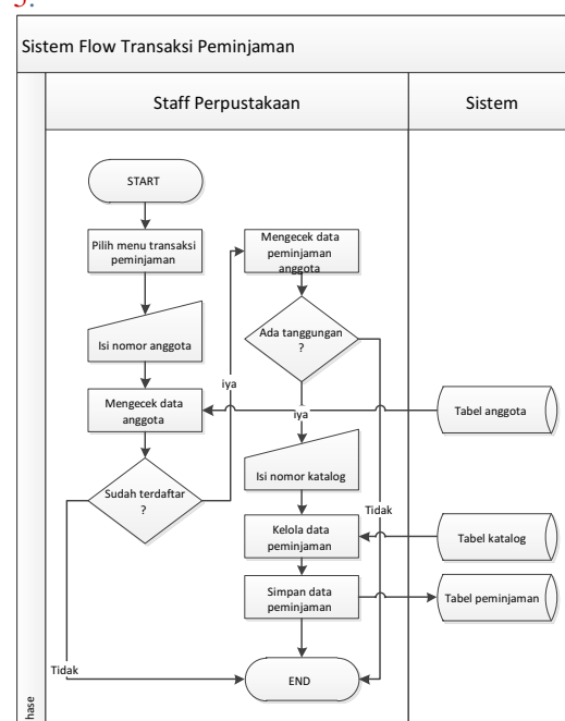
Gambar 5 System Flow Transaksi Peminjaman
