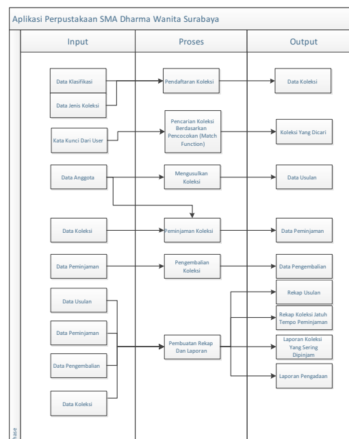
Gambar 2 Block Diagram Sistem Informasi Perpustakaan SMA Dharma Wanita Surabaya
