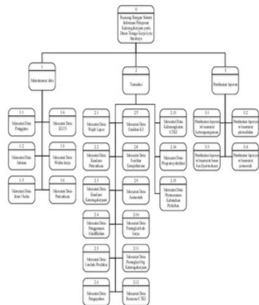
Gambar 2 Diagram HIPO
