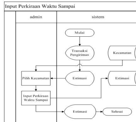
Gambar 5. System Flow Input Perkiraan Waktu Sampai
