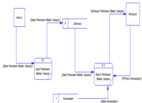
Gambar 12. DFD level 1 Perkiraan Waktu Sampai
