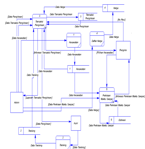
Gambar 10. DFD Jasa Pengiriman
