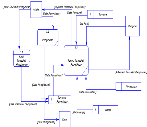
Gambar 11. DFD level 1 Transaksi Pengiriman
