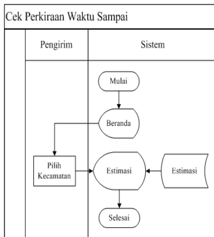
Gambar 8. System Flow Cek Perkiraan Waktu Sampai
