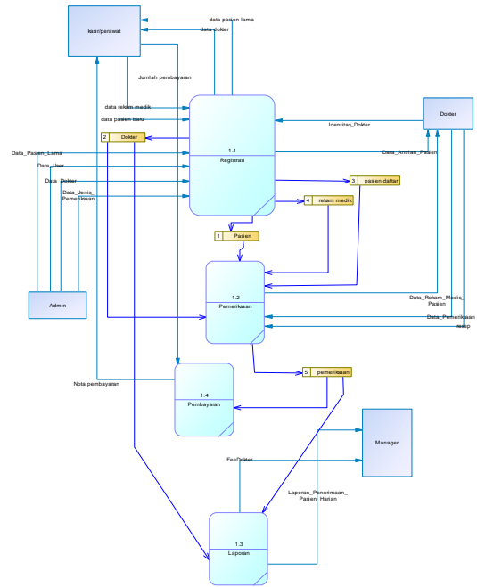
DFD Level 0
